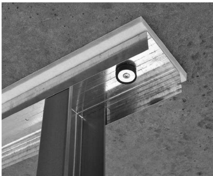
Монтаж звукоизоляционной перегородки с применением звукоизолирующего направляющего профиля Vibrofix Liner 100
